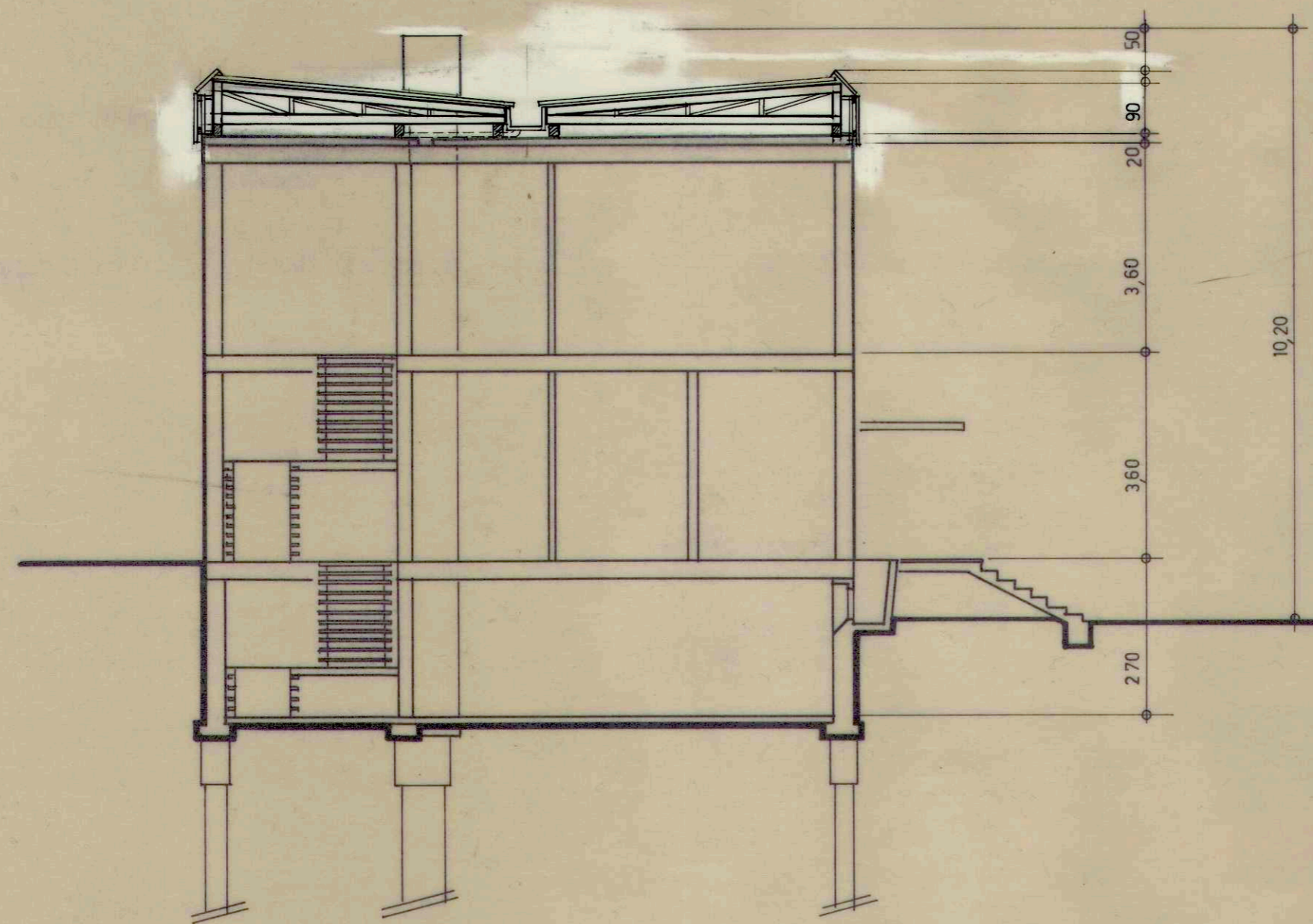
QUERSCHNITT
